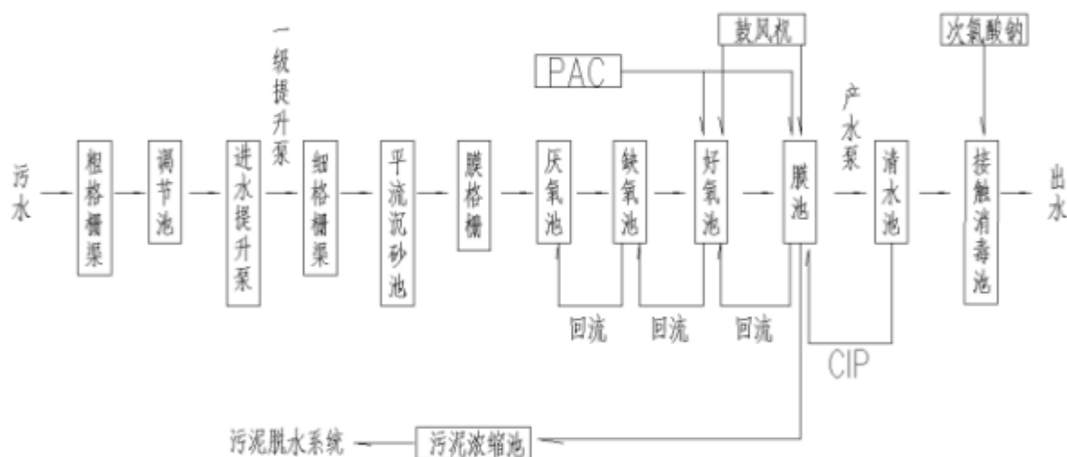
图3.5-1 污水处理工艺流程图
