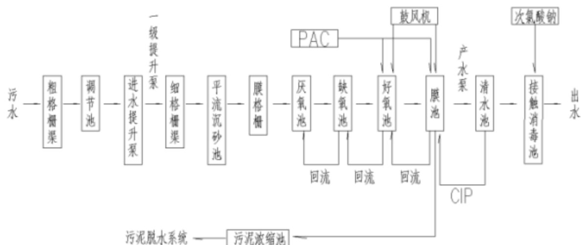
图3.6-1 污水处理工艺流程图
