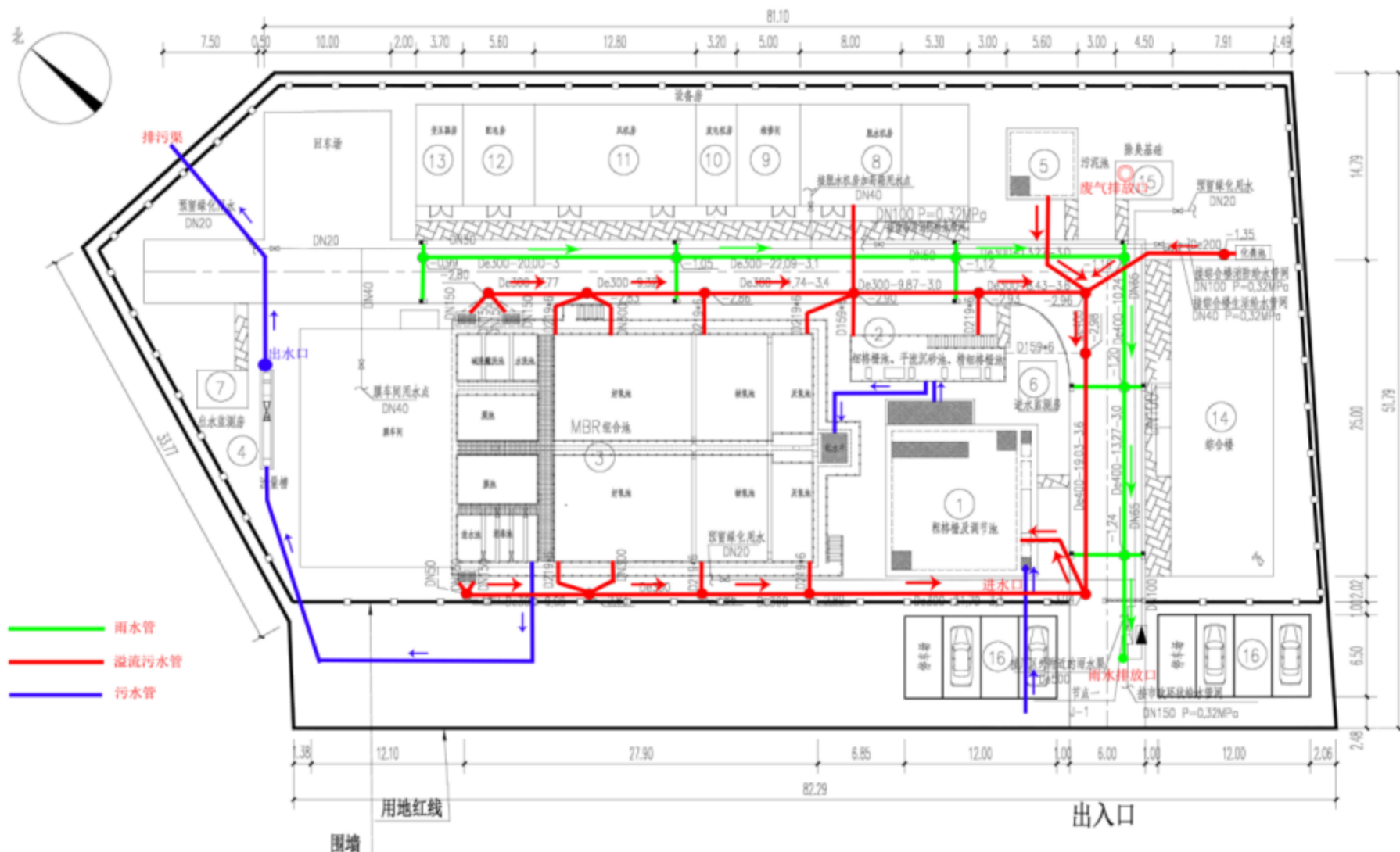
3.1-5 厂区平面布置图
