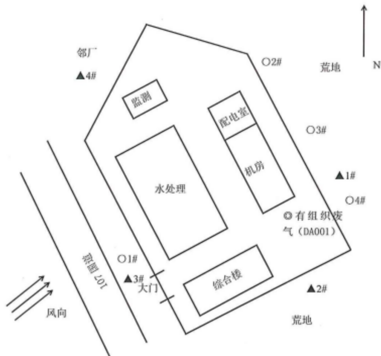
附图 1: 检测布点图, “▲”表示噪声检测点位, “◎”表示有组织废气检测点位 “○”表示无组织废气检测点位。
