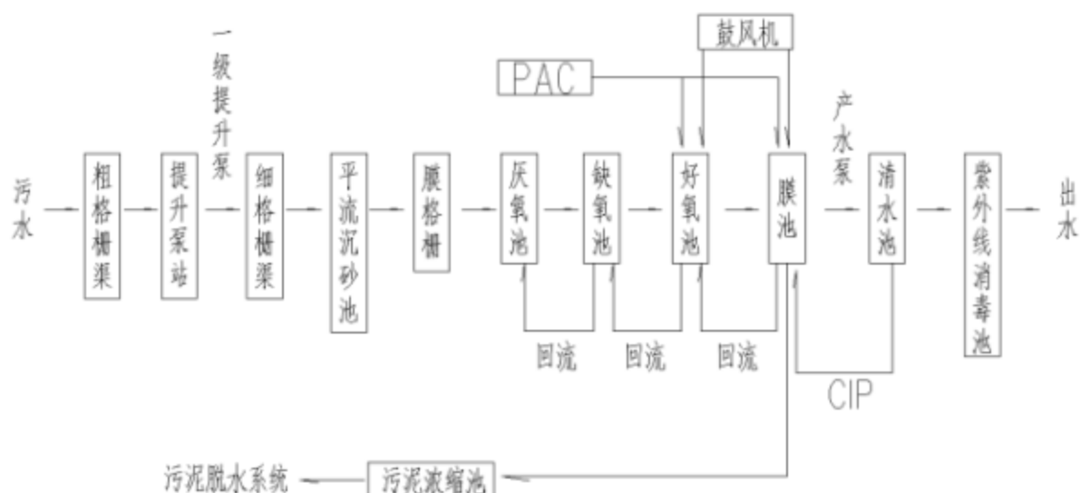
图3.6-1 污水处理工艺流程图
