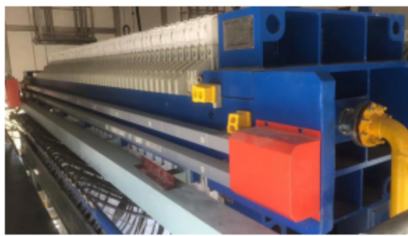
板框压滤机
