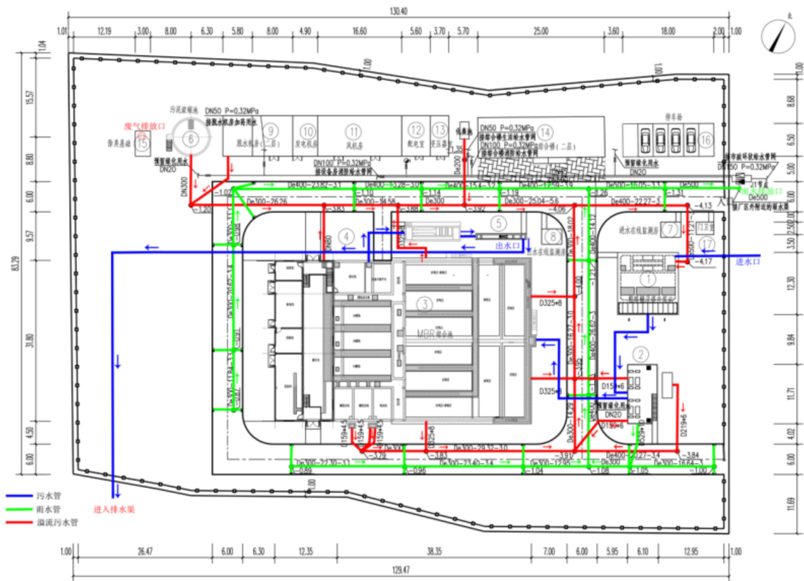
3.1-5 厂区平面布置图
