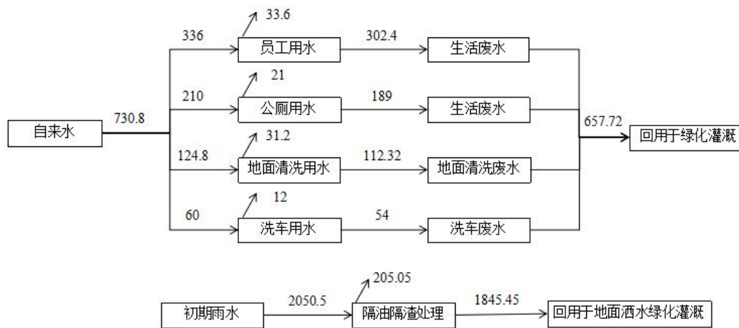
图 3.4-1 项目水平衡图 (单位: \text{m}^3/\text{a} )
