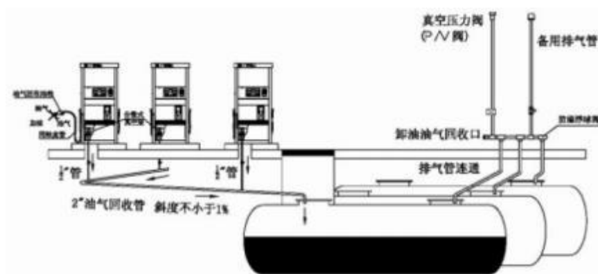
图 4.1-2 分散式油气回收系统工艺流程图
