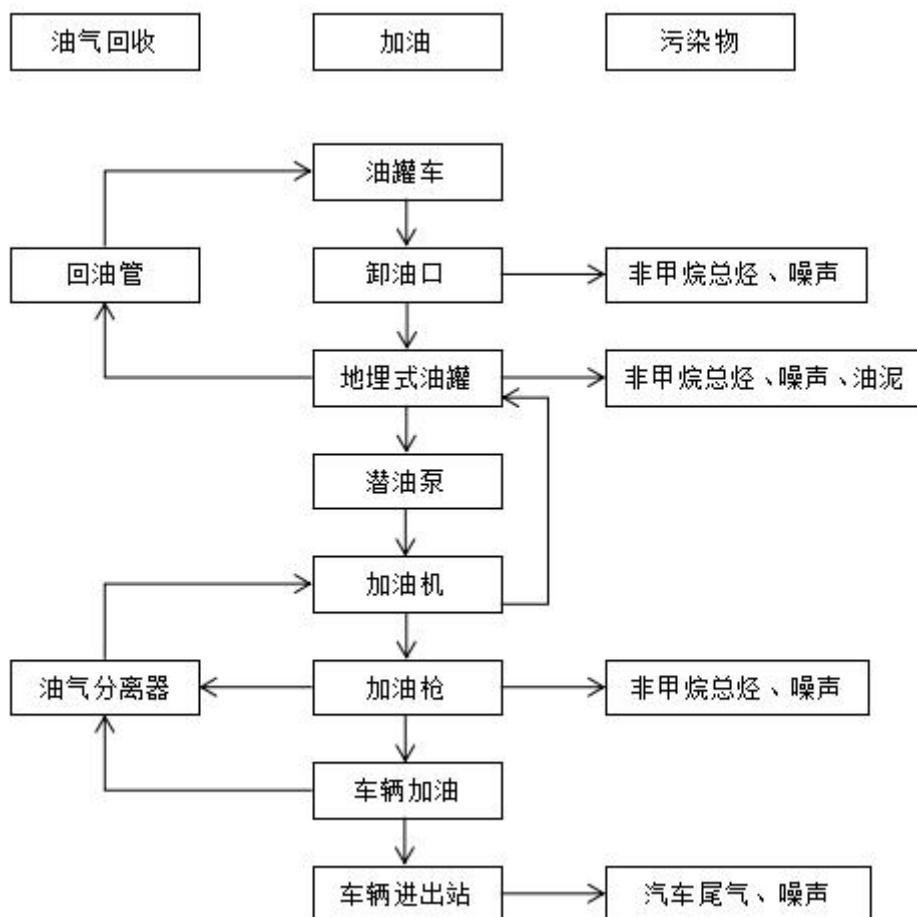
图 3.5-1 加油工艺流程及产排污环节图
