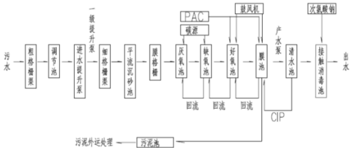
图3.6-1 生产工艺流程图
